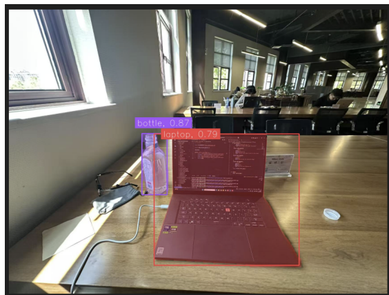
(b) YOLOE-11M
