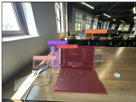
(d) YOLOE-v8L
